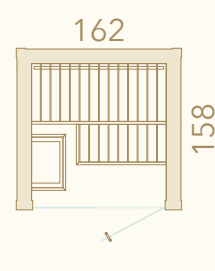
Mira S con esterno in abete termotrattato, naturale
